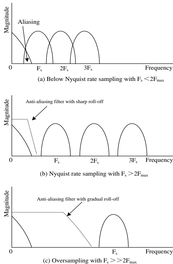
图 2.2 过采样技术放宽了对模拟抗混叠滤波器的要求
