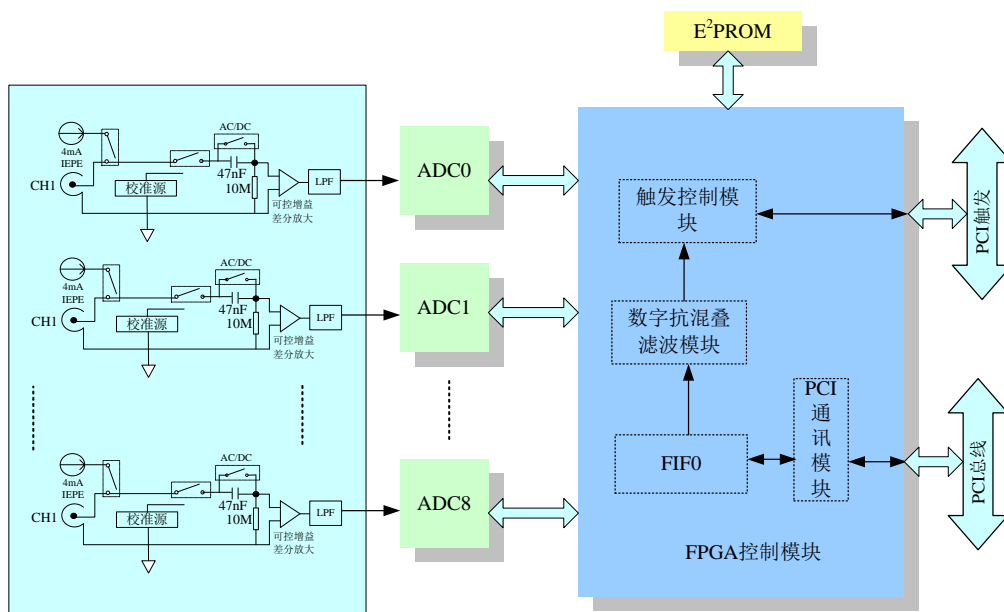
图 1.2 系统框图
