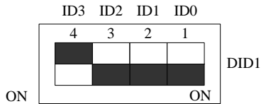
图二 表示“0111”，则代表的物理ID号为7
