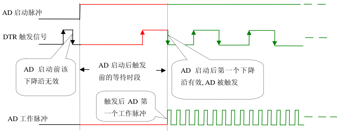
图 6.2 下降沿触发图例
